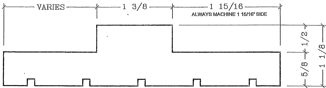
DOUBLE RABBET JAMB
