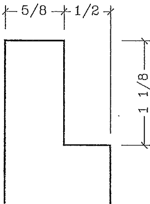
SIDE JAMB RABBET
